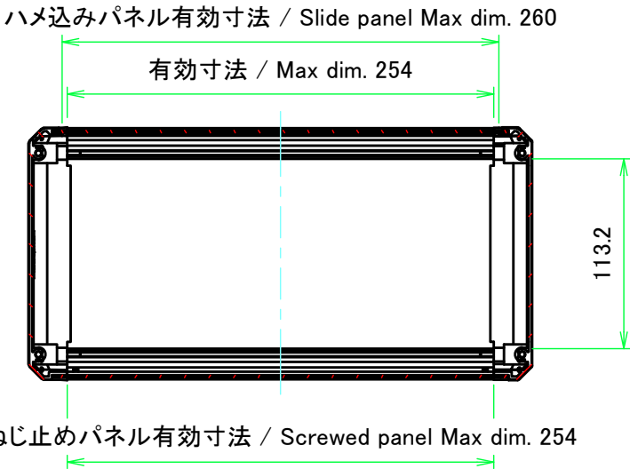
A-A ( 1 : 4 )
