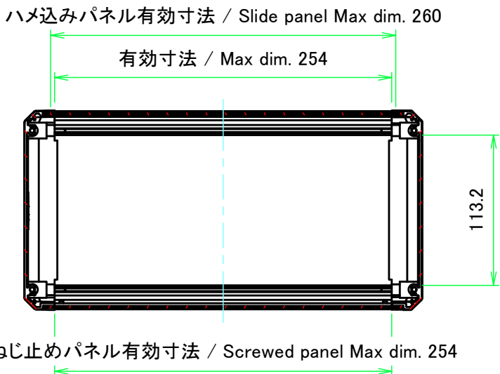
A-A ( 1 : 4 )
