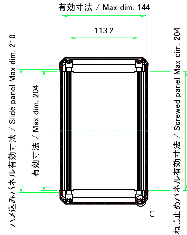
B-B ( 1 : 4 )
