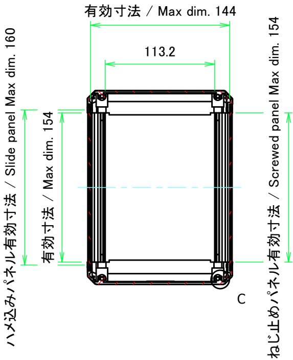
B-B ( 1 : 4 )
