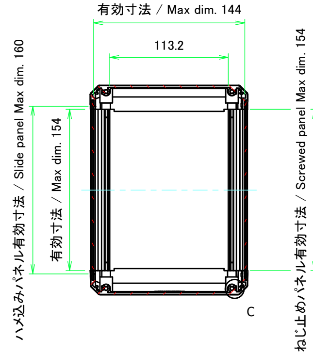
B-B ( 1 : 3.5 )
