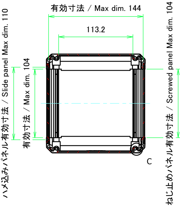
B-B ( 1 : 3.5 )
