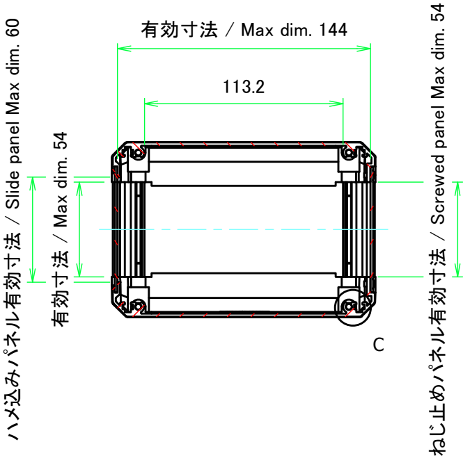
B-B ( 1 : 3 )
