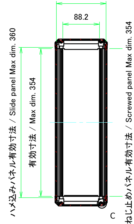
B-B ( 1 : 5.5 )
