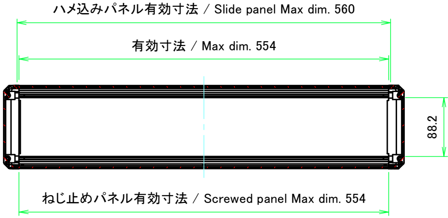
A-A ( 1 : 5.5 )
