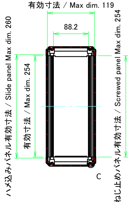
B-B ( 1 : 5.5 )
