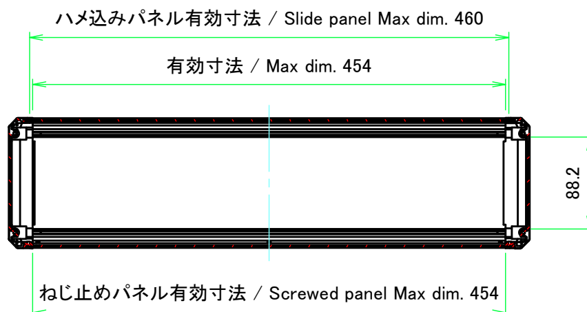
A-A ( 1 : 5 )
