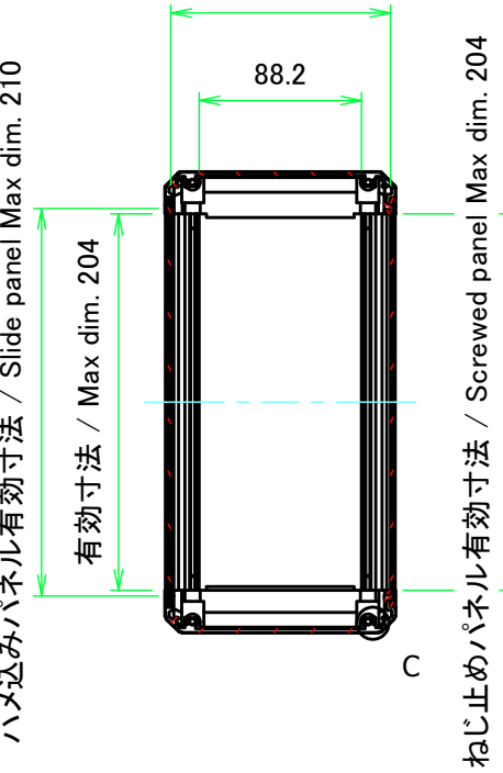
有効寸法 / Max dim. 119
