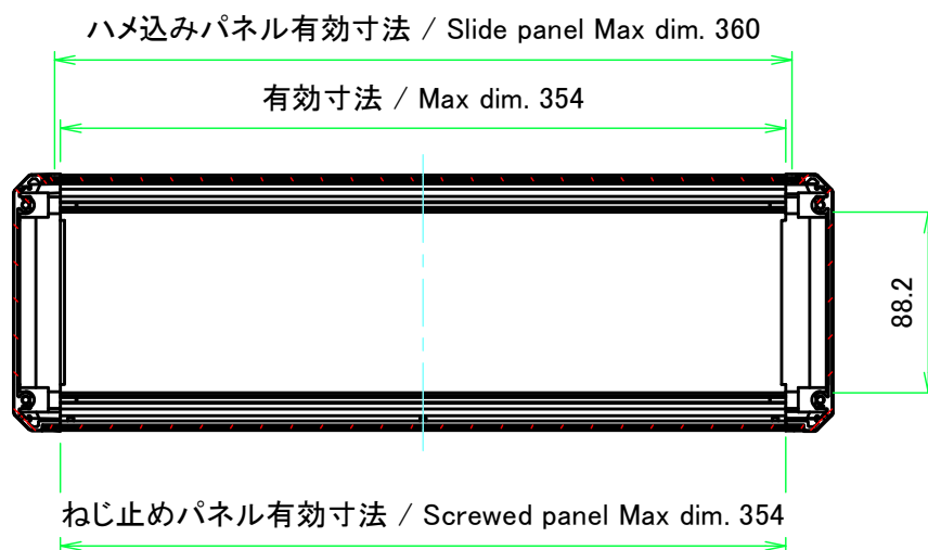
A-A ( 1 : 4 )
