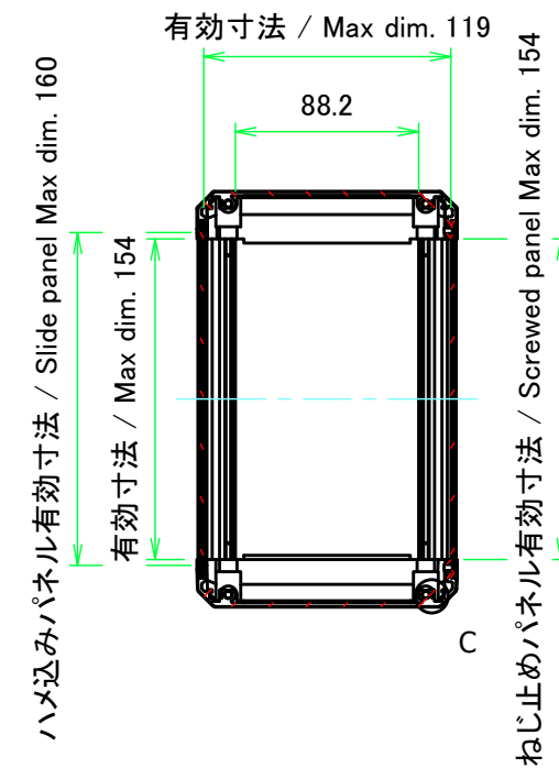
B-B ( 1 : 4 )
