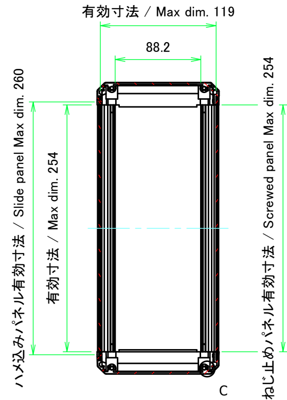
C : フレーム拡大図 / Frame cross-section
