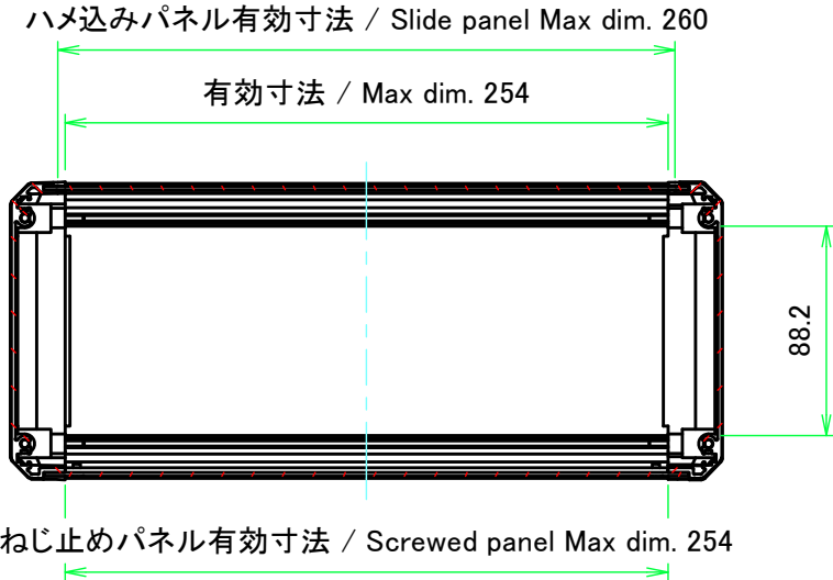
A-A ( 1 : 3.5 )
