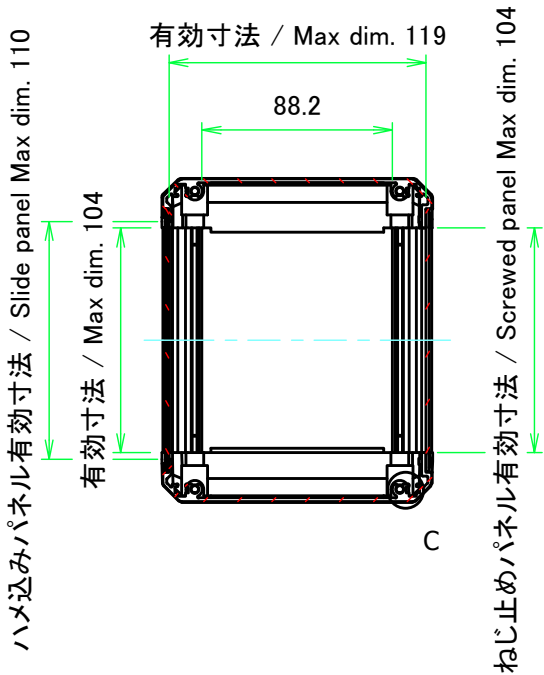
B-B ( 1 : 3.5 )
