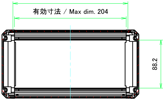
A-A ( 1 : 3.5 )
