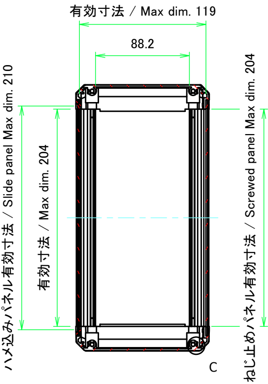
B-B ( 1 : 3.5 )
