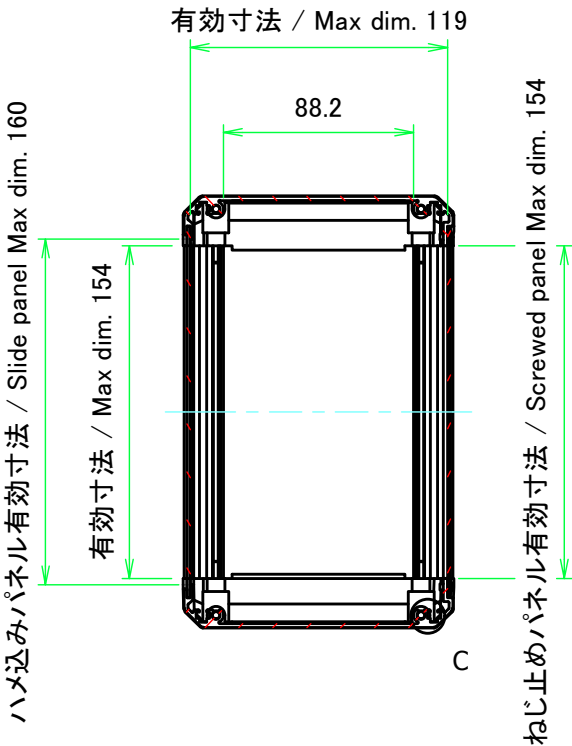
B-B ( 1 : 3.5 )
