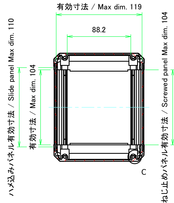
B-B ( 1 : 3 )
