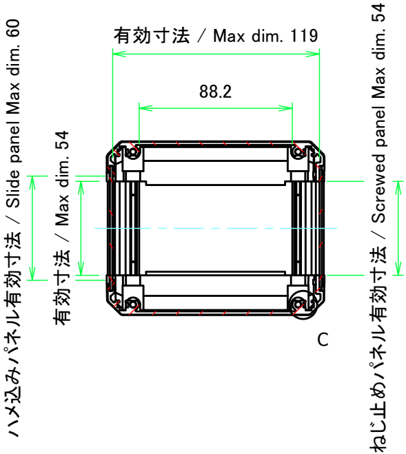
B-B ( 1 : 3 )
