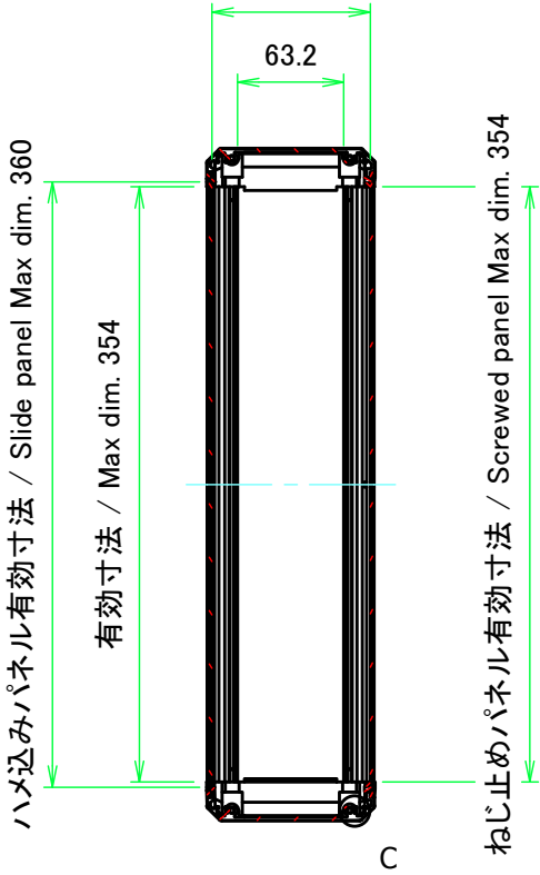
B-B ( 1 : 5 )
