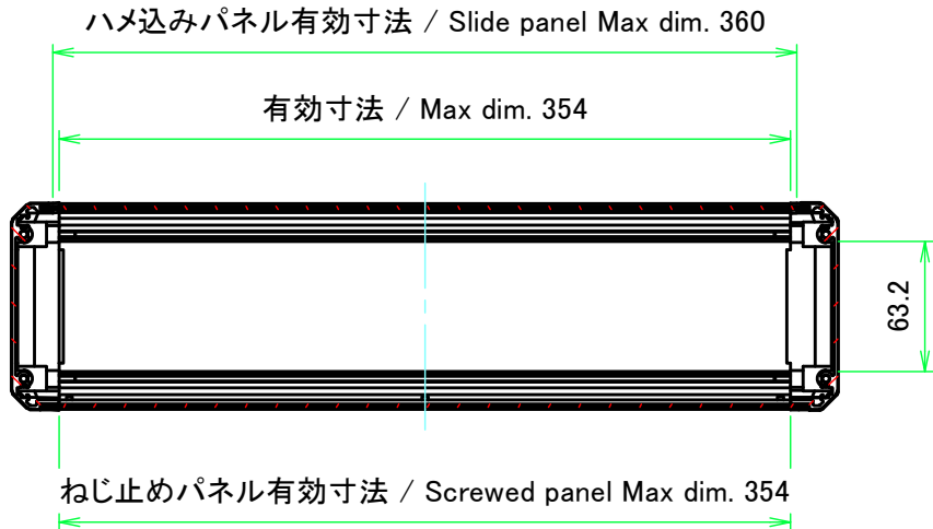
A-A ( 1 : 4 )
