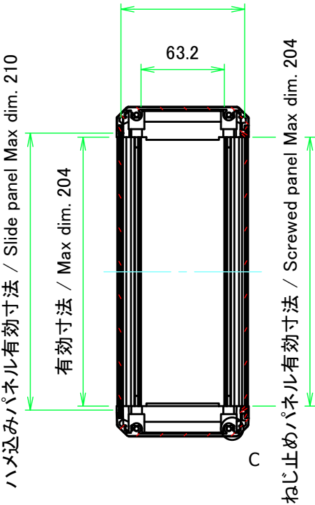
B-B ( 1 : 4 )
