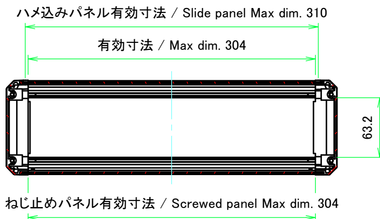
A-A ( 1 : 4 )
