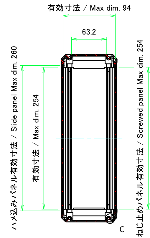
B-B ( 1 : 4 )
