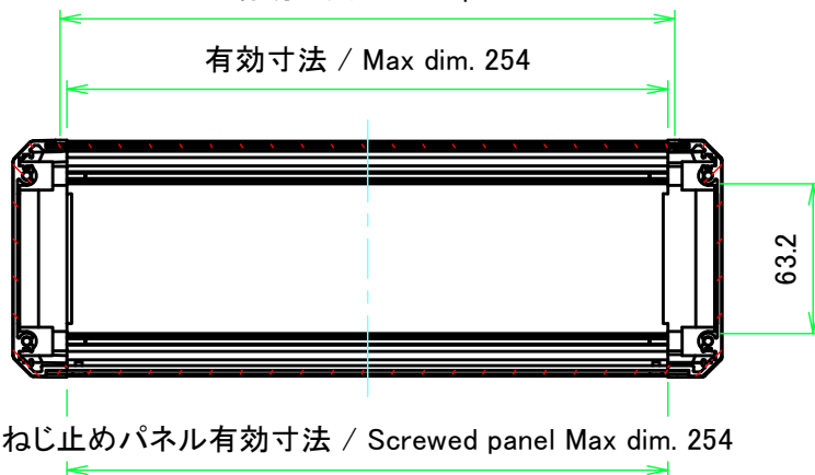
A-A ( 1 : 3.5 )
