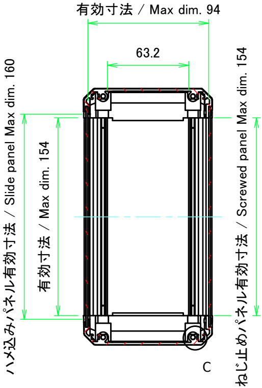
B-B ( 1 : 3 )
