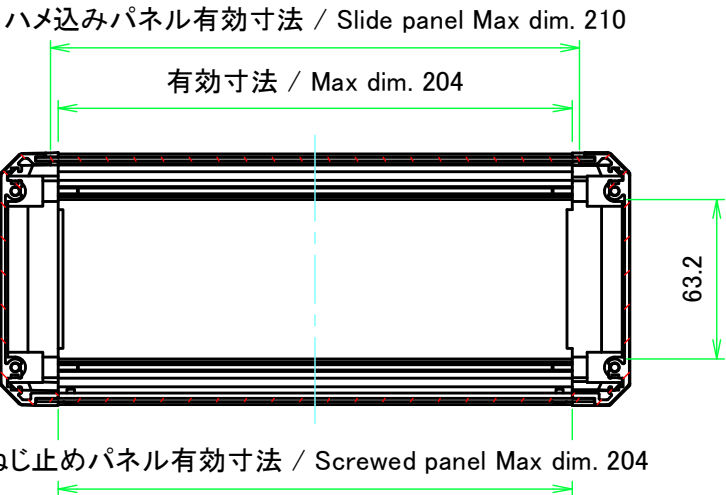
A-A ( 1 : 3 )
