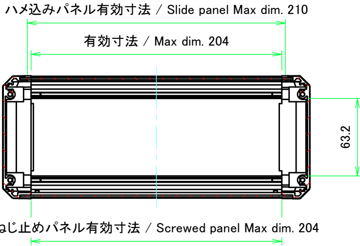
A-A ( 1 : 3 )
