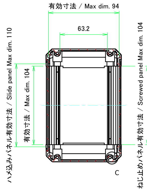
B-B ( 1 : 2.5 )
