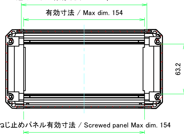
A-A ( 1 : 2.5 )
