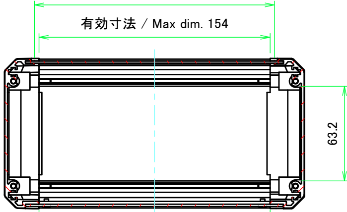
A-A ( 1 : 2.5 )
