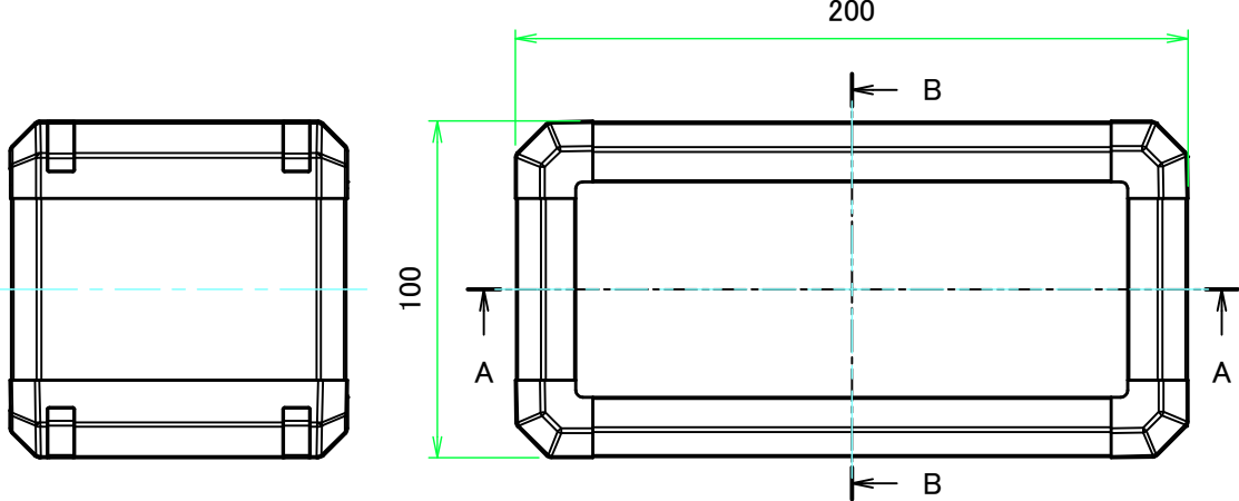
フレーム2側 / Frame2 side
