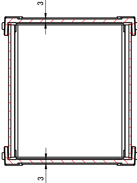
D-D (1:2)
