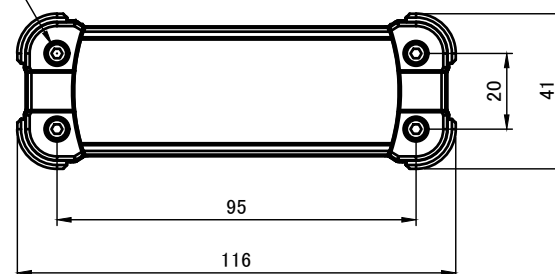
A-A (1:2)
