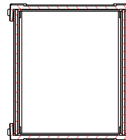
C-C (1:2)
