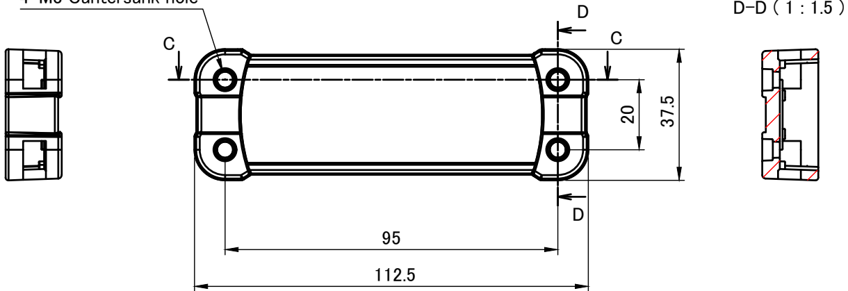
D-D ( 1 : 1.5 )
