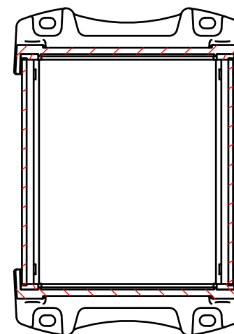
D-D (1:2)
