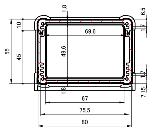
A-A (1:2)
