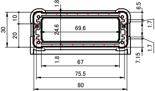
A-A ( 1 : 2 )
