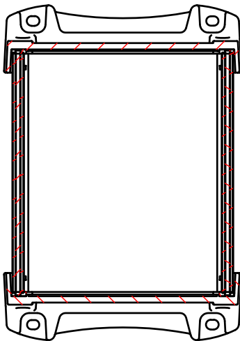
D-D ( 1 : 2.5 )
