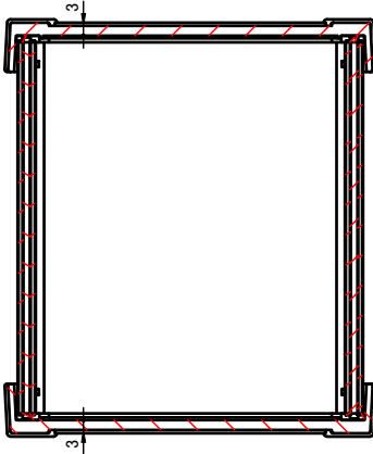
C-C ( 1 : 2.5 )
