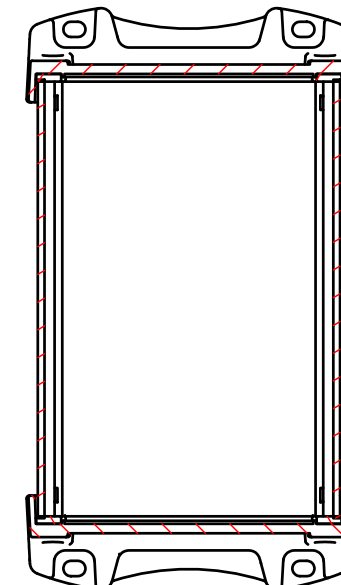
D-D (1:2)
