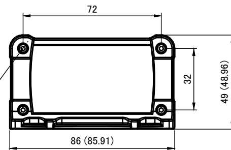
A-A (1:2)
