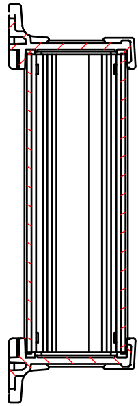
B-B (1:2)
