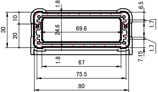
A-A ( 1 : 2 )
