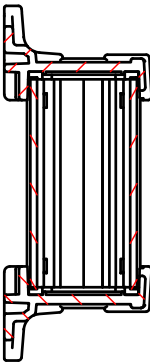
B-B ( 1 : 2 )
