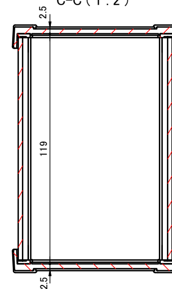
C-C (1:2)
