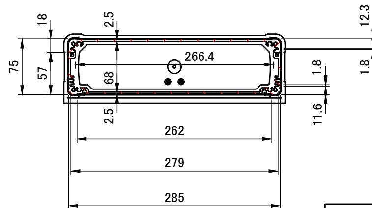
A-A (1:5)
