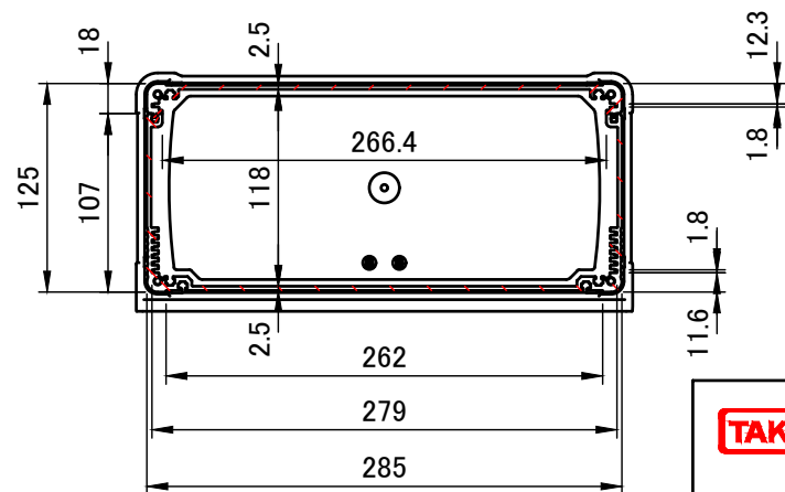
A-A (1:5)
