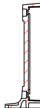
D-D (1:3)
