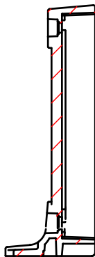
D-D (1:3)
