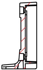
D-D (1:3)
