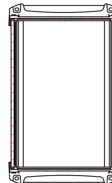
D-D (1:5)
