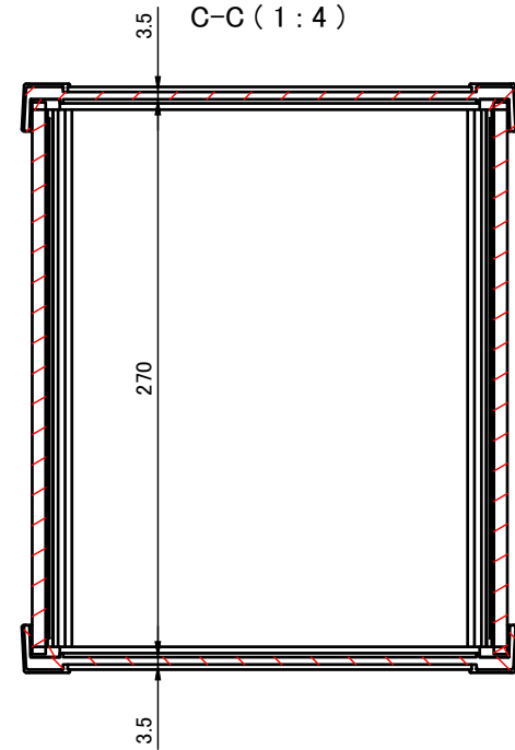
C-C ( 1 : 4 )
