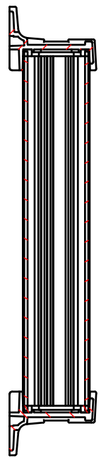
B-B ( 1 : 4 )
