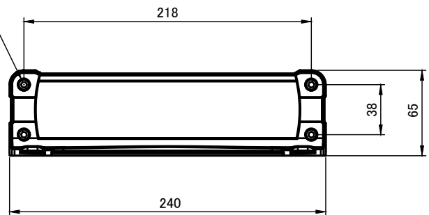
A-A ( 1 : 4 )
