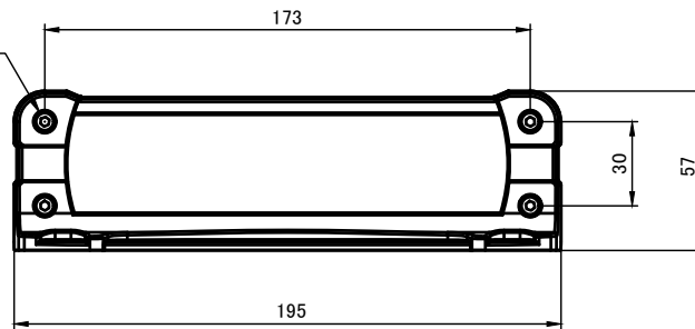
A-A (1:3)
