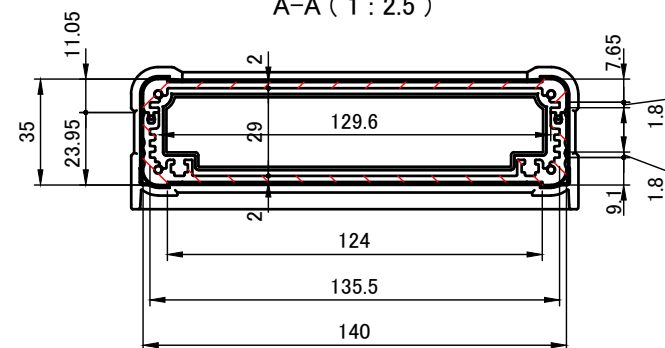
A-A (1:2.5)
