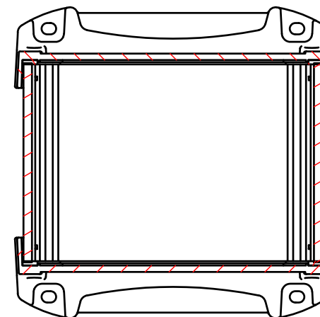
D-D (1:2.5)
