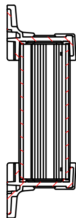
B-B (1:2.5)
