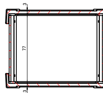
C-C ( 1 : 2.5 )
