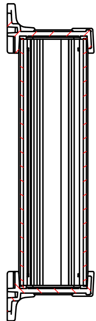
B-B (1:2.5)
