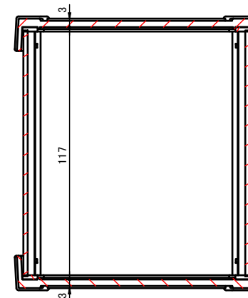
C-C ( 1 : 2.5 )
