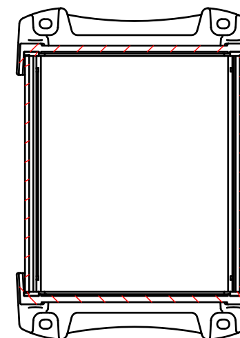
D-D ( 1 : 2.5 )
