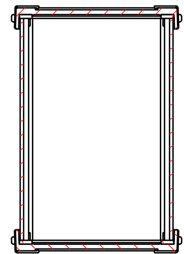
C-C (1:2)
