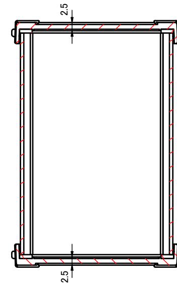
D-D (1:2)
