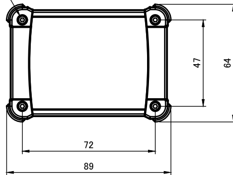
A-A (1:2)
