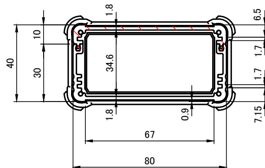
A-A (1:2)
