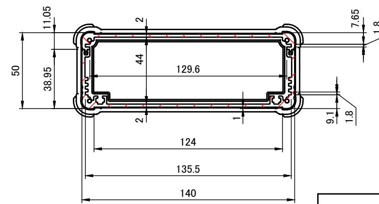
A-A ( 1 : 2.5 )
