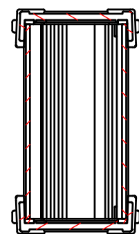
B-B ( 1 : 2.5 )
