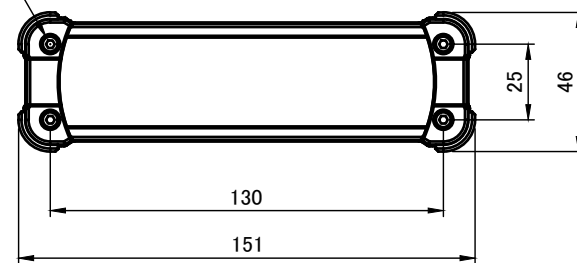
A-A ( 1 : 2.5 )
