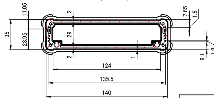
A-A ( 1 : 2.5 )
