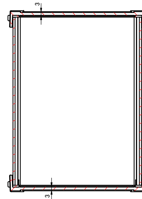
D-D ( 1 : 2.5 )
